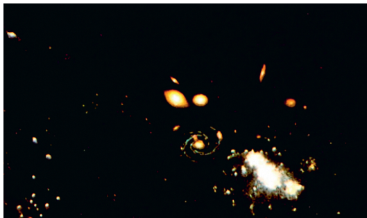
Более крупное скопление, включающее неправильную галактику (справа внизу). Художники А. Шеллер и Р. Стернбах
