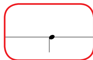
Четвертная нота
