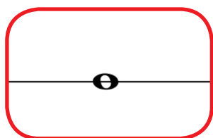
Целая нота
