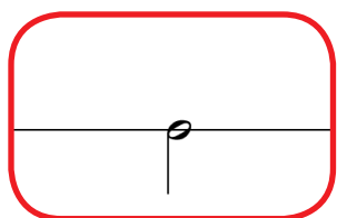
Половинная нота
