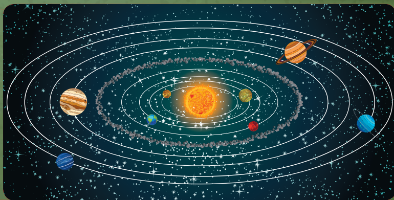
Солнечная система.
