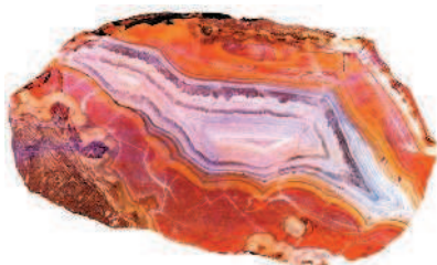
Срез окрашенного агата
