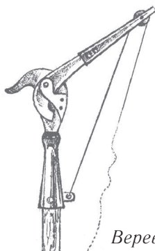
Рычажный сучкорез
