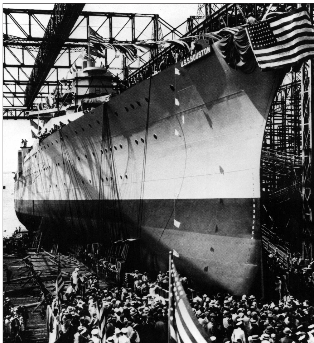
Готовый к спуску со стапеля «Хьюстон», 7 сентября 1929 г.
