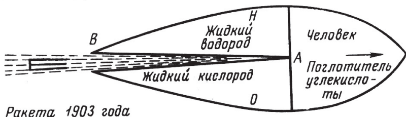
Схема ракеты с прямой дюзой Константина Циолковского (1903)
