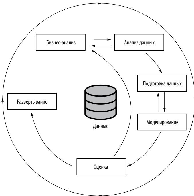
Рис. 1.9. Процесс CRISP-DM. Проект машинного обучения начинается с понимания проблемы, а затем переходит к подготовке данных, обучению модели и оценке результатов. Наконец модель добирается до этапа развертывания. Процесс является итеративным, и на каждом шаге можно вернуться к предыдущему
