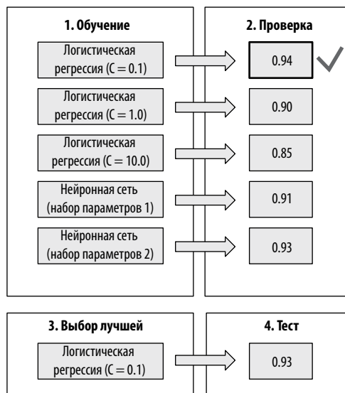
Рис. 1.14. Использование тестового набора данных для подтверждения того, что производительность наилучшей модели на проверочном наборе является хорошей
