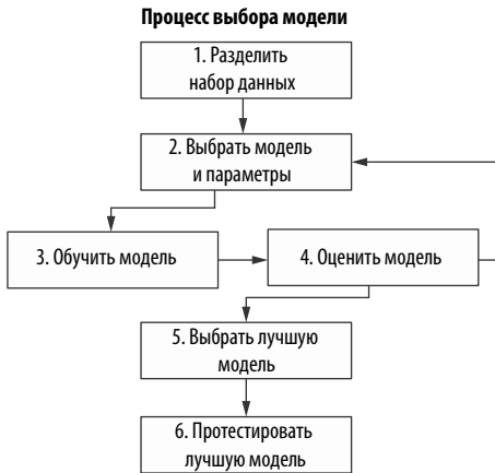
Рис. 1.15. Сначала мы разбиваем набор данных, выбираем модель и обучаем ее только на обучающей части данных. Затем, на этапе проверки, мы оцениваем модель. Мы повторяем этот процесс многократно, пока не обнаружим лучшую модель
