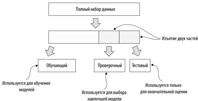
Рис. 1.13. Разделение данных на обучающую, тестовую и проверочную части
