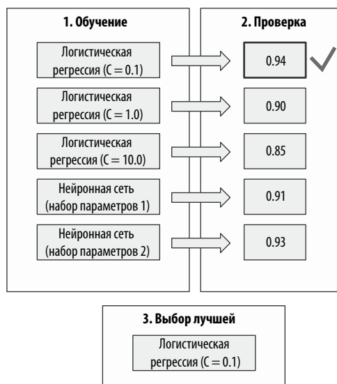
Рис. 1.12. Использование проверочного набора данных для выбора наилучшей модели с наилучшими параметрами
