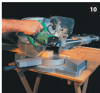
Торцовочно-усорезная дисковая пила с протяжкой обеспечивает максимальные возможности пиления среди всех электрических торцовочных пил. Двигатель перемещается к оператору, затем опускается на заготовку и режет в процессе возврата в исходное положение.
