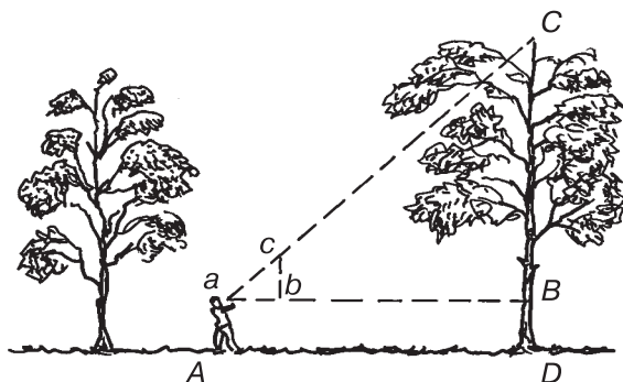
Рис. 5. Схема применения булавочного прибора
