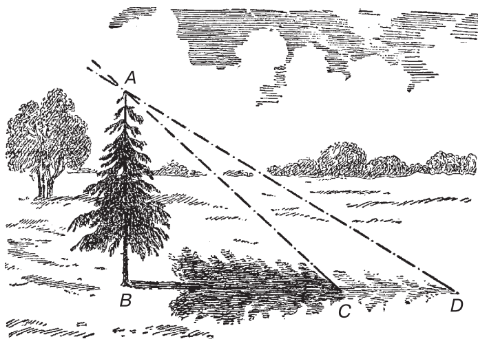
Рис. 3. Как образуется полутень
