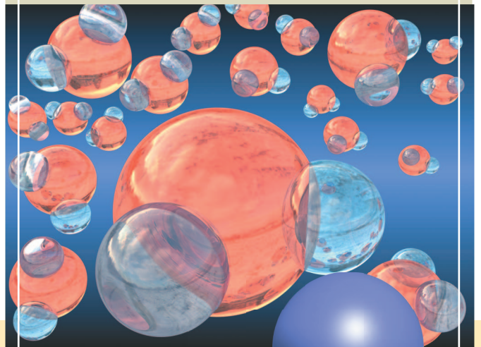
Молекулы воды.
