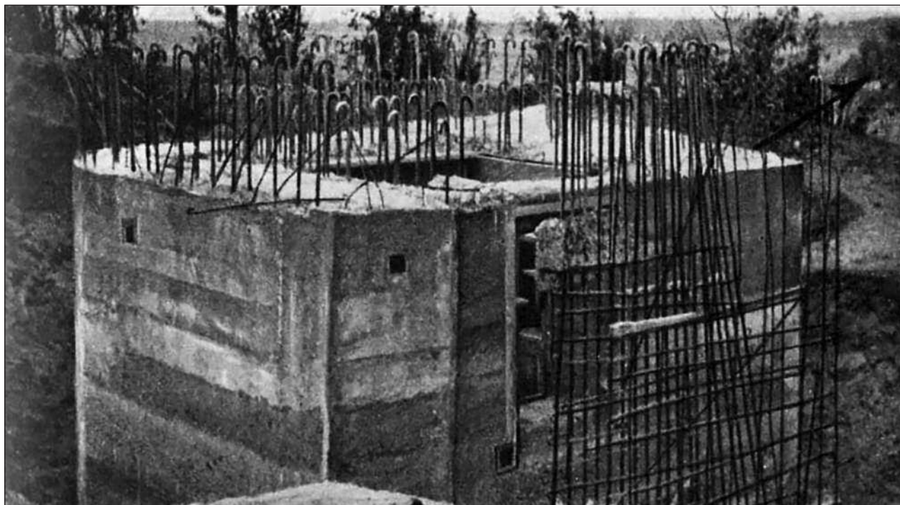
Возведение ДОТа
