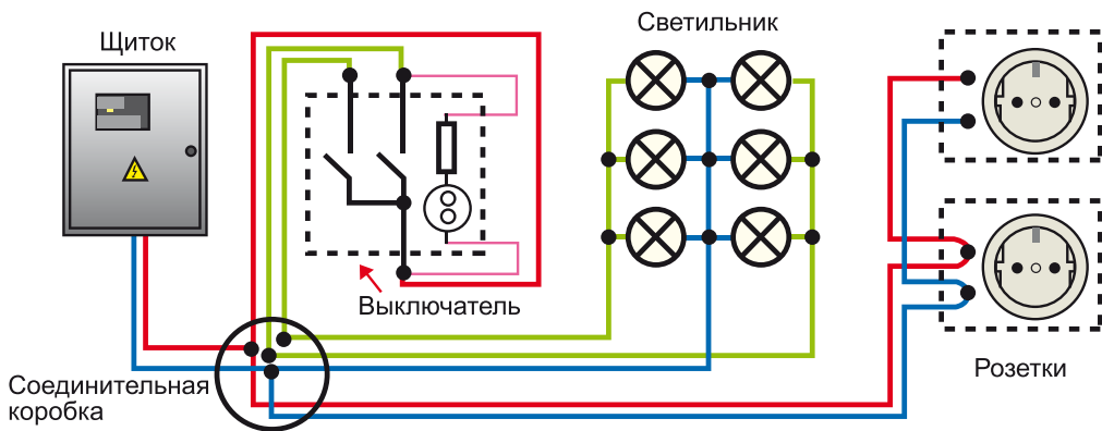
Рис. 9.4. Простейшая схема розеток, выключателей и ламп
