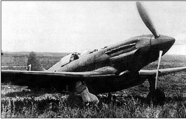
Истребитель МиГ-3 на полевом аэродроме. «Миги» к началу войны были самым массовым истребителем нового типа
