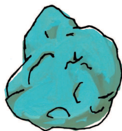
БИРЮЗА
