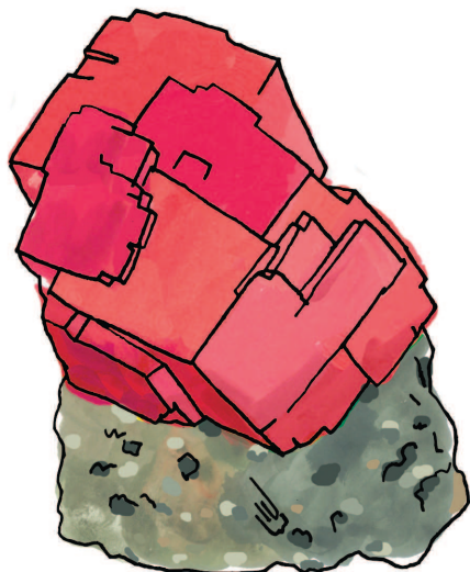
РОДОХРОЗИТ
