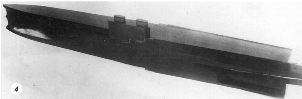
4 — вариант с одним островом по левому борту; 5 — разработанный для «Фьюриеса» вариант с островом по правому борту (не был принят, но послужил основой при переоборудовании однотипных «Глориеса» и «Корейджеса»); 6 — проект оснащения «Виндиктива» сплошной полетной палубой и островом по правому борту; 7 — проект «Игла» со сплошной полетной палубой без надстроек (апрель 1918 г.)
