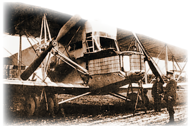
Бомбардировщик R.I фирмы «Сименс». На этой фотографии хорошо видны приводные валы, идущие от моторов, установленные в фюзеляже к воздушным винтам
