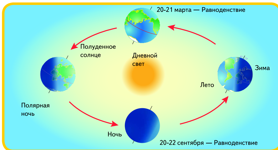
▲ Схема, поясняющая механизм возникновения белых ночей (полярных дней).
