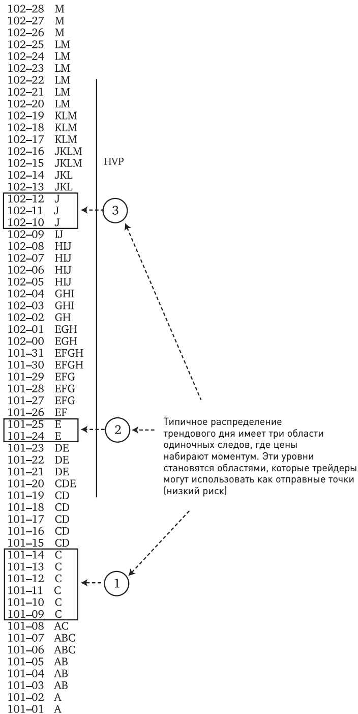
Рис. В. 5. Распределение трендового дня
