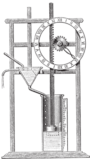
Рис. 4. Водяные часы.
