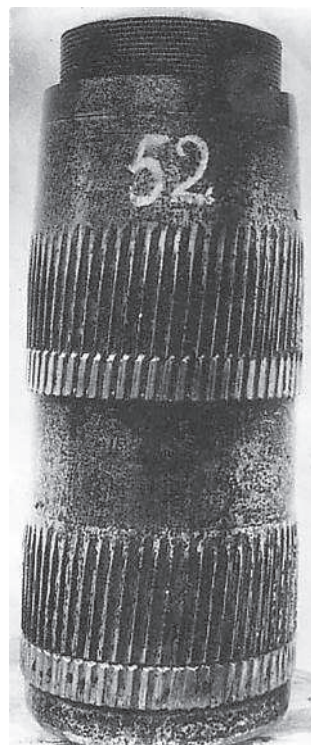
Из истории «нарезных» снарядов. Снаряды германской 21-см сверхдальнобойной пушки «Колоссаль» (1918 г.) имели два ведущих пояска с готовыми нарезками. На фото — снаряд без баллистического колпачка
