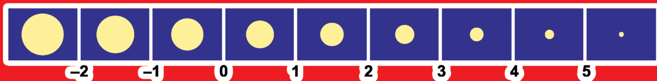
Распределение звездных величин.
