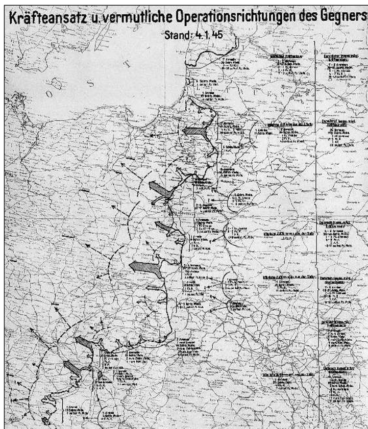
Представление немецкой разведки о планах советского командования по состоянию на 5 января 1945 г. Размер стрелки пропорционален силе предполагаемого удара
