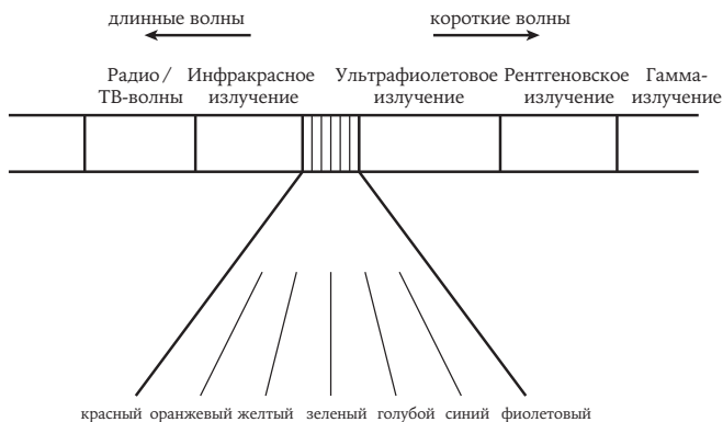
Рис. 4. Бóльшая часть электромагнитного спектра, простирающегося от радио- до гамма-излучения, невидима для наших глаз. Из-за размера клеток в сетчатке наши глаза способны различать лишь крохотную часть электромагнитного спектра
