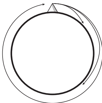
Рис. 1. Если стрелять так, чтобы пушечное ядро получало раз от раза все большую энергию, то в конечном итоге оно обогнет Землю и вернется в начальную точку. Затем Ньютон сказал, что этим объясняется и траектория движения Луны, объединив таким образом физические законы Земли с законами движения небесных тел
