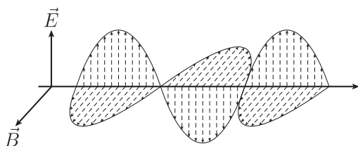
Рис. 3. Электрическое и магнитное поля — две стороны одной медали. Переменные электрическое и магнитное поля превращаются одно в другое и движутся подобно волне. Свет — одно из проявлений электромагнитной волны
