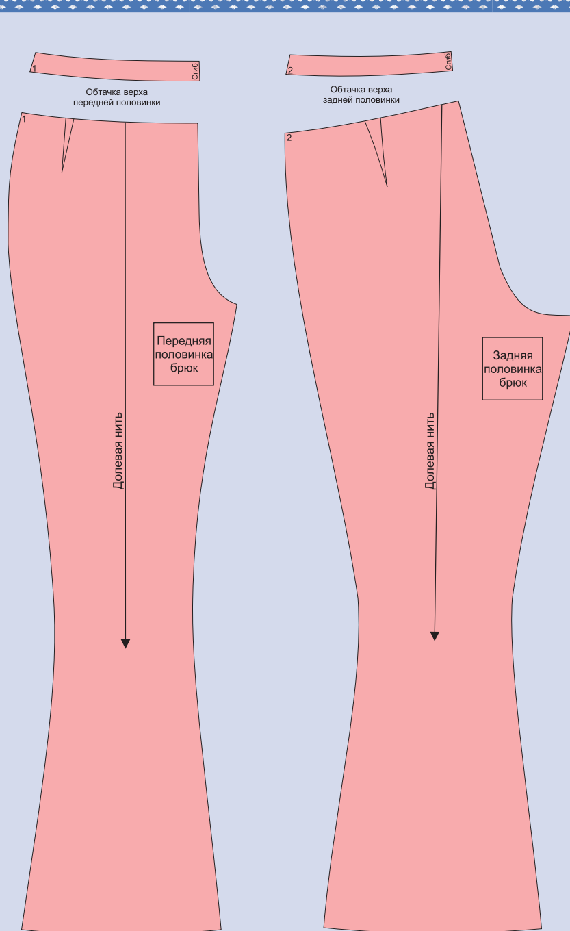
Детали выкройки брюк
