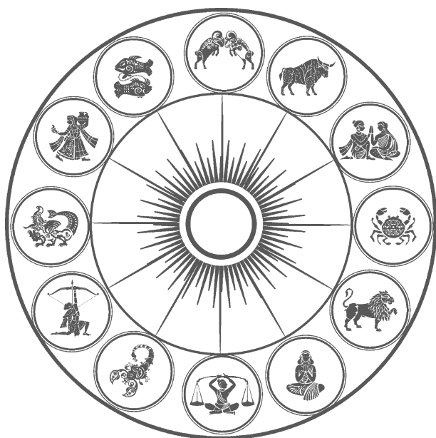
Рис. 1. Зодиакальный круг
