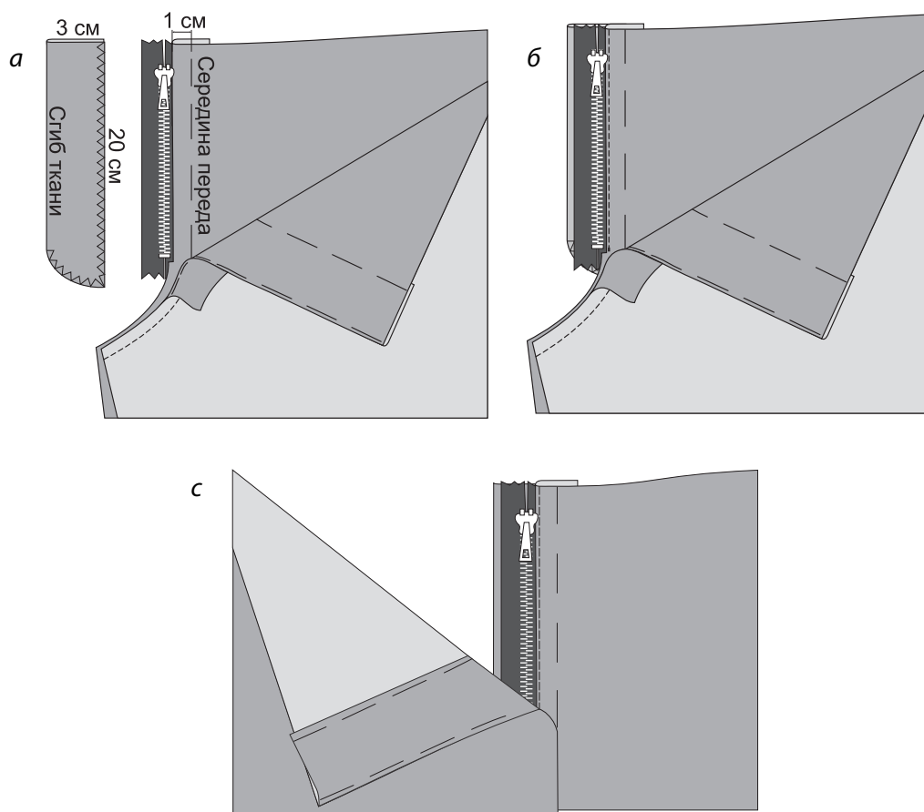
Рис. 1. Технология обработки застежки-молнии с цельнокроеным подзором
