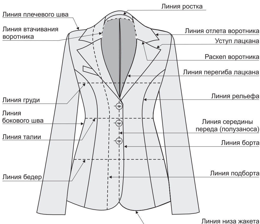
Рис. 269. Контрольные линии жакета
