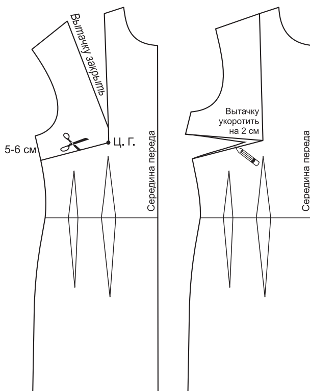
Рис. 131. Перевод нагрудной вытачки на линию бока
