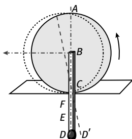
Рис. 8. Опыт с кружочком и спичкой. Когда колесо откатывается налево, точки F , E , D выступающей части спички подвигаются в обратную сторону.
