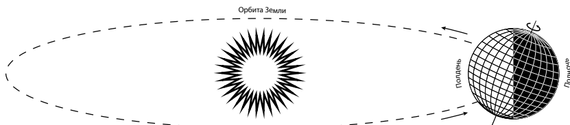
Рис. 6. На ночной половине земного шара люди движутся вокруг Солнца быстрее, чем на дневной.
