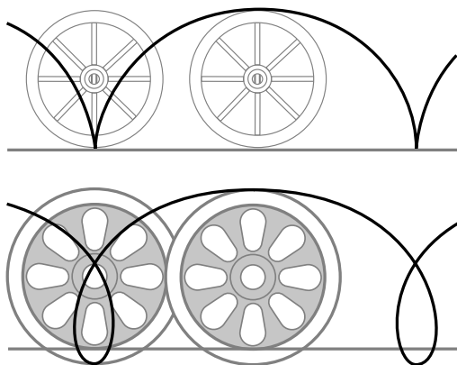
Рис. 10. Вверху изображена та кривая линия («циклоида»), которую описывает каждая точка обода катящегося колеса телеги. Внизу — кривая линия, описываемая каждой точкой выступающего края железнодорожного колеса.
