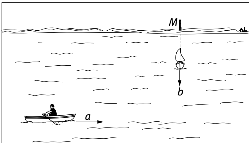
Рис. 11. Парусная лодка идет наперез весельной. Стрелки a и b — скорости. Что увидят гребцы?
