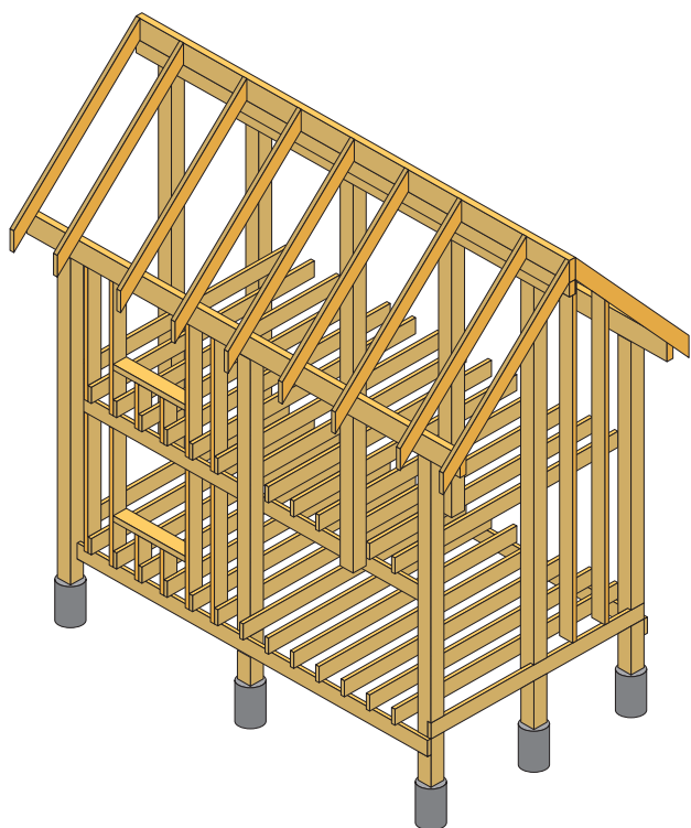
Рис. 1.6. Каркас стоечной конструкции
