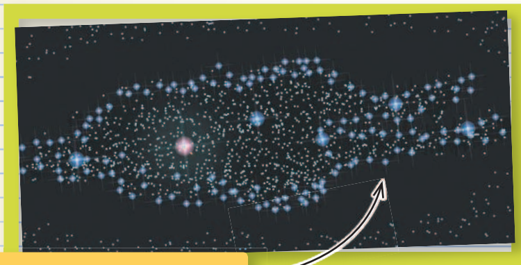
Млечный Путь (вид сверху).
