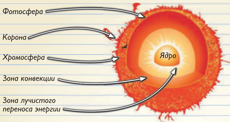
Внутреннее строение Солнца.
