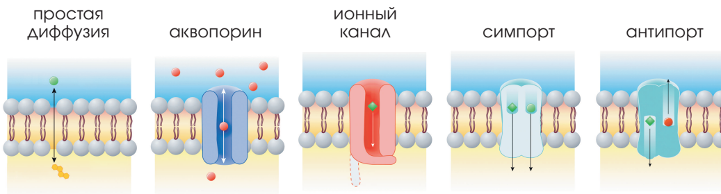
Мембранный транспорт
