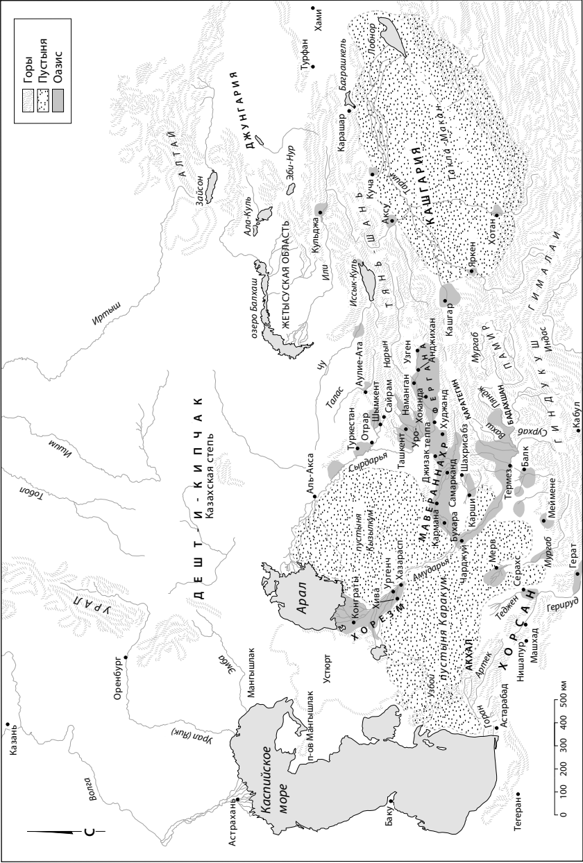
Карта 0.2. Центральная Азия: особенности физической географии и исторические географические названия
